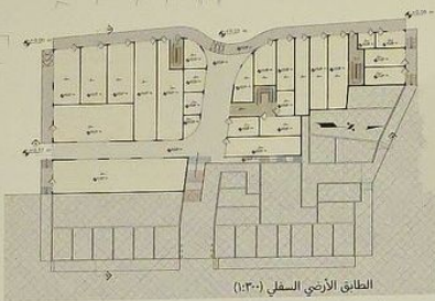
الطابق الأرضي السفلي (١:٣٠٠)
