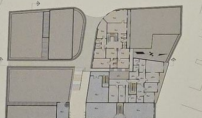
الطابق الثالث (١:٣٠٠)
