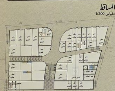
المسقط الأفقي للطابق السفلي الأول
