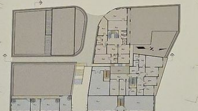
الطابق الثاني (١:٣٠٠)
